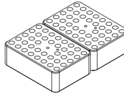
Typ HB-BIO1 L/B/H 140 x 98 x 46 mm 38 Epp.gefäße 1,5 ml
