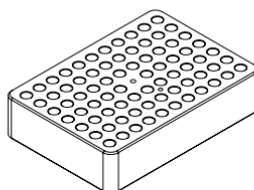
Typ HB-BIO2 L/B/H 198 x 140 x 46 mm 96 Epp.gefäße 1,5 ml
