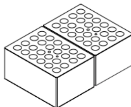
Typ HB-EC1 L/B/H 148 x107 x75 mm 24 Rea.gläser Ø 16 mm
