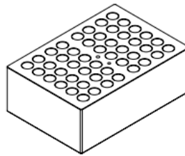
Typ HB-EC2 L/B/H 214 x 148 x 75 mm 48 Rea.gläser Ø 16 mm
